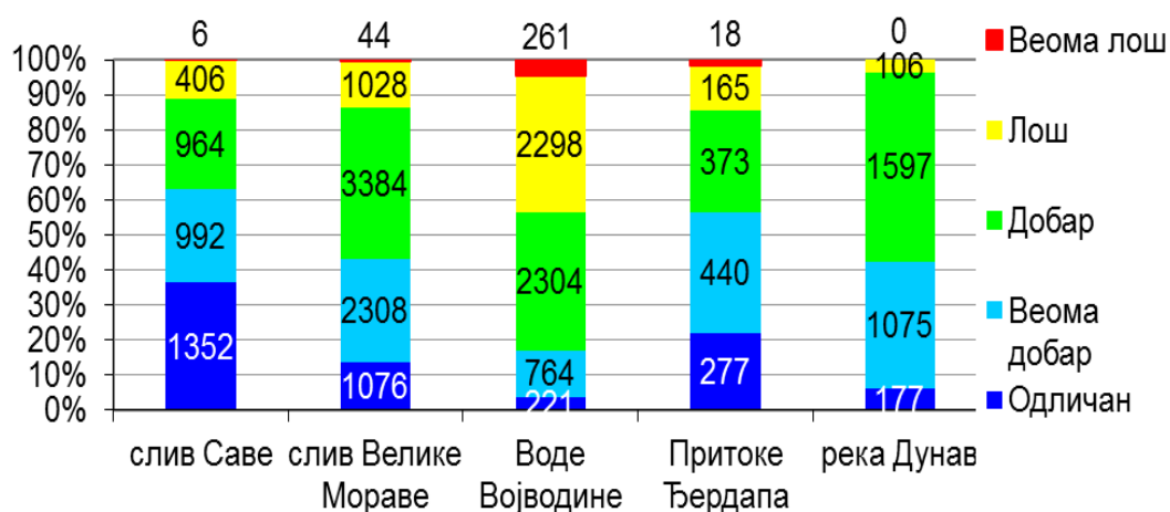
Слика 36. Процент квалитета свих узорака воде по сливовима (са одговарајућим бројем узорака) за период 1998-2013. година одређених методом SWQI
