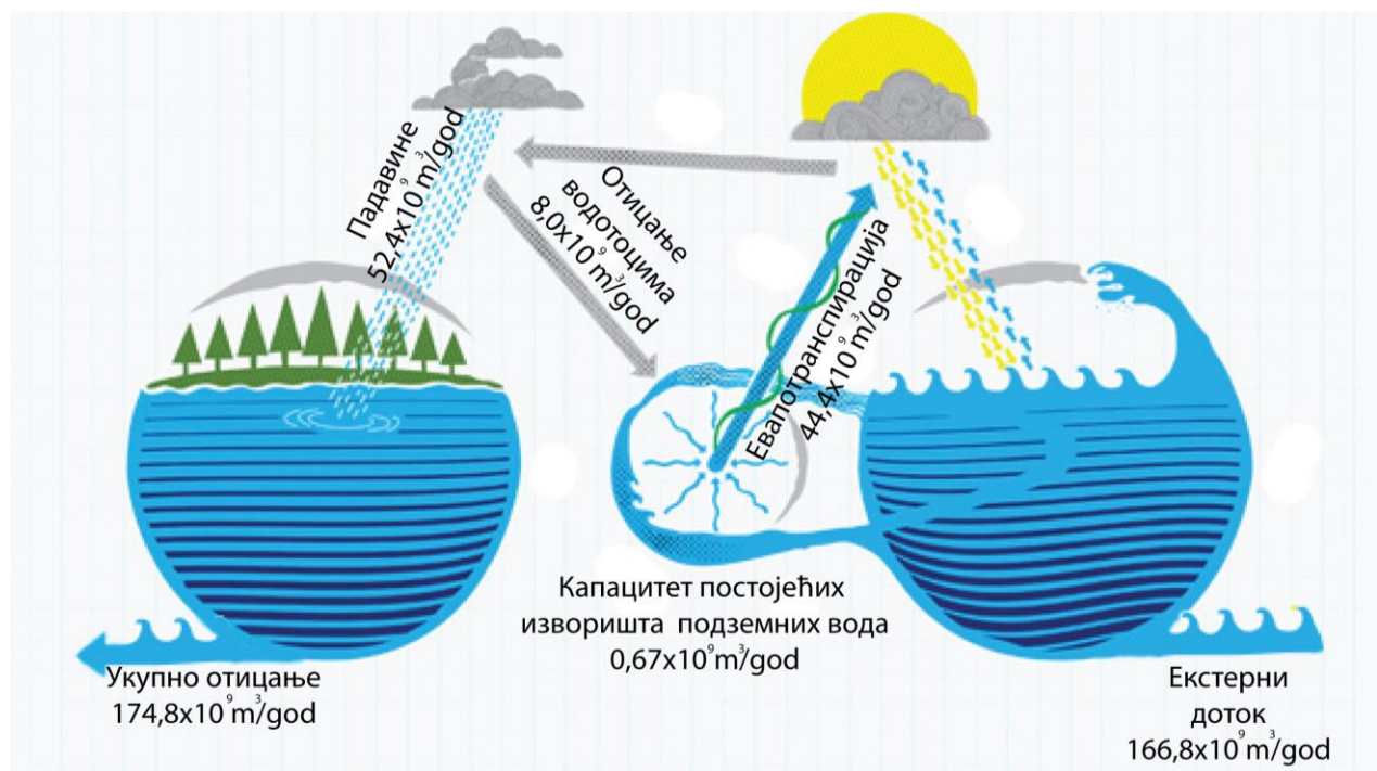
Слика 12. Биланс вода Републике Србије (2000-2011)
