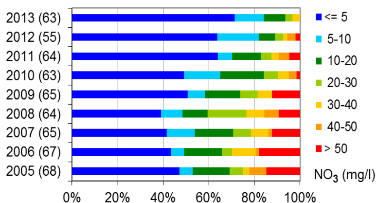
Слика 49. Расподела учесталости концентрација нитрата (2005-2013)
