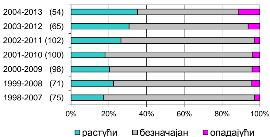
Слика 41. Процентуална заступљеност врсте тренда SWQI на мерним местима по декадама
