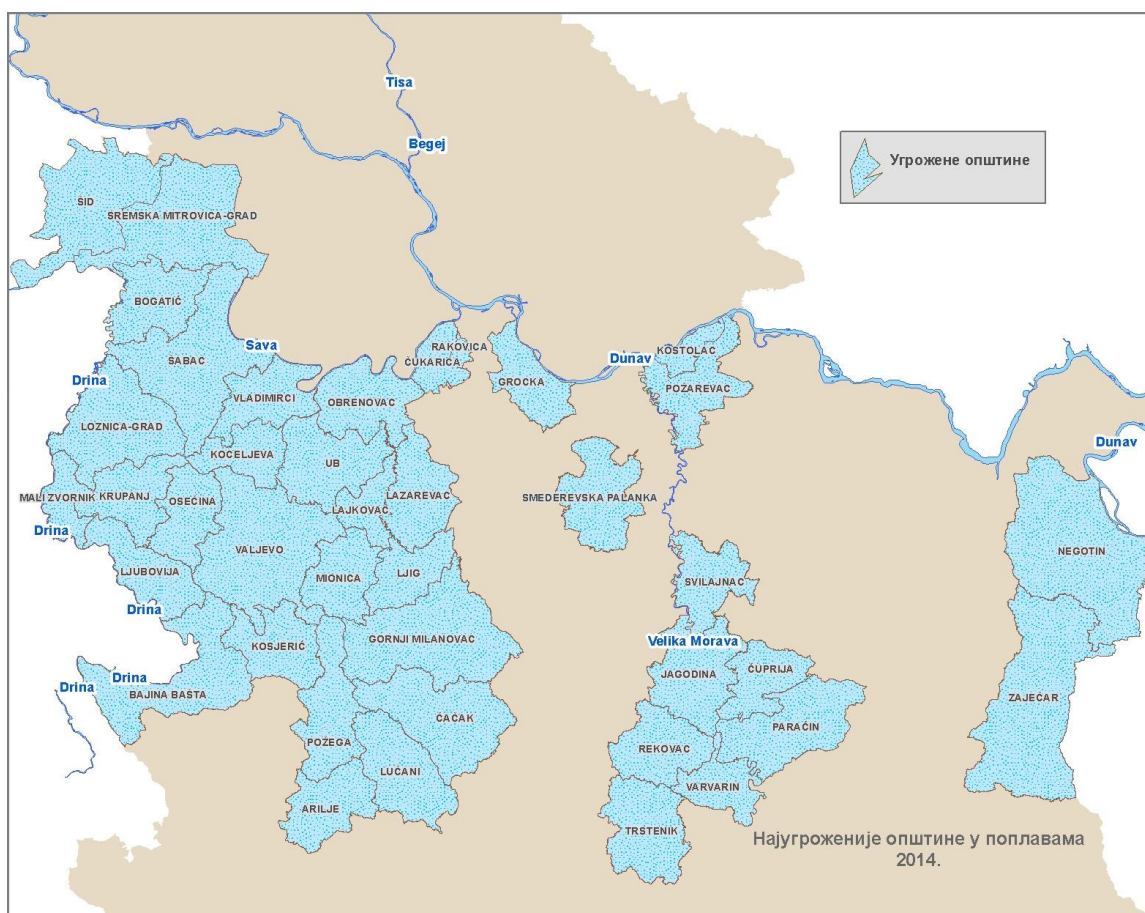
Слика 57. Најугроженије општине у поплавама маја 2014. у Републици Србији (Извештај, 2014) 22
