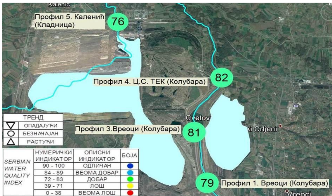
Слика 88. Просечне вредности индикатора SWQI – Зона 1; период 25.09. – 21. 10.2014.
