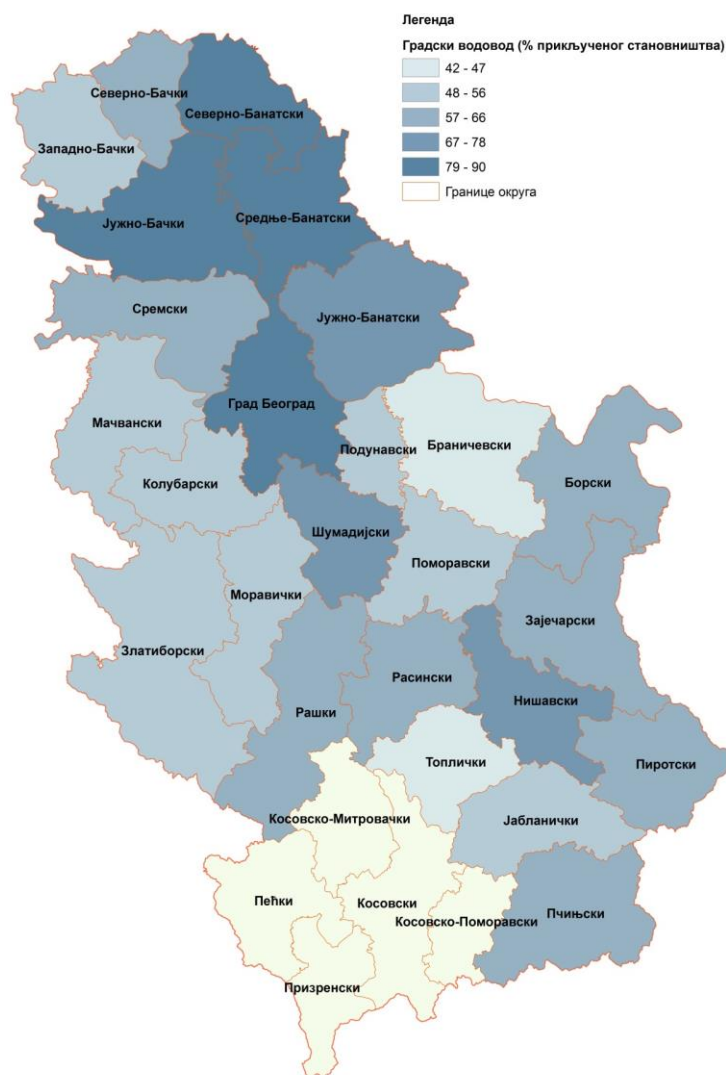
Слика 22. Процент становника прикључен на системе јавног водоснабдевања
